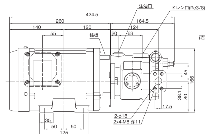
HBPP-3BH4※-VB2V-8A※-B(-G) (サイドポート形)
