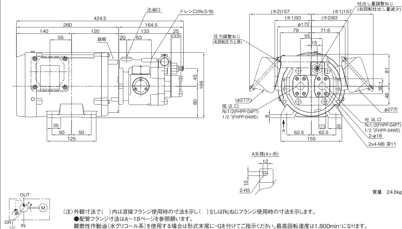
HBPP-3※4-VB2V-8A※-EE-B(-G) (アキシャルポート形)
