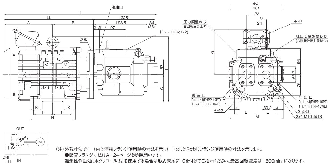
HBPP-3※4-VD2V-31A※-EE-B(-G) (アキシャルポート形)
