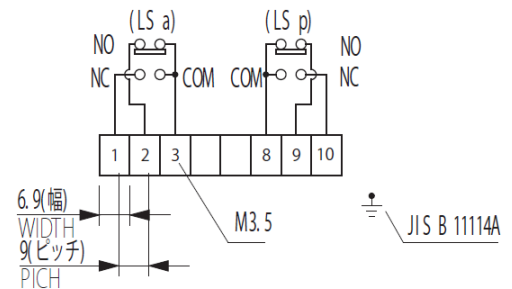
端子台配線図 TERMINAL WIRING
